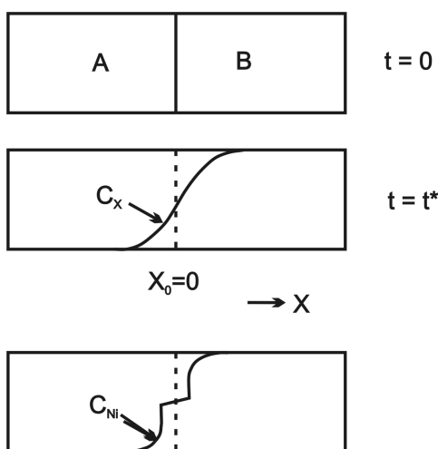
3.ábra • Koncentráció-eloszlás diffúziós párban ha szilárdoldat keletkezik (középső ábra), vagy ha új fázis növekszik (alsó ábra).
