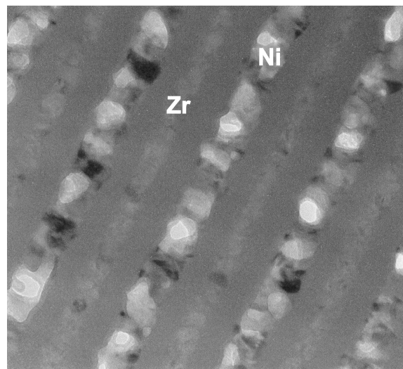
4.ábra • Amorf NiZr fázis keletkezik szilárdtest reakcióban nanokristályos Ni/Zr multirétegekben (300 °C-on, 4 óra)
