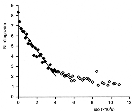
8. ábra • A Ni film Auger elektronspektroszkóp segítségével meghatározott vastagságának időbeli változása. Kezdetben 8 atomi réteg vastagságú film volt a Cu mátrixon, melynek vastagsága időben lineárisan csökken.
