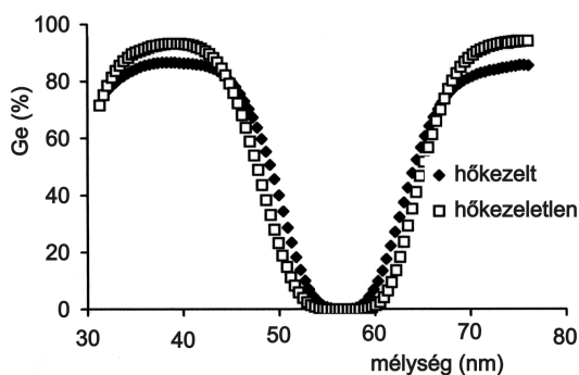
6. ábra • Hőkezletlen, illetve hőkezelt amorf Si/Ge multirétegek Auger mélységi profilja. Látható, hogy a hőkezelt minta esetében a Ge réteg Si-mal töltődött és megvastagodott, miközben a Si réteg tiszta maradt és elvékonyodott.
