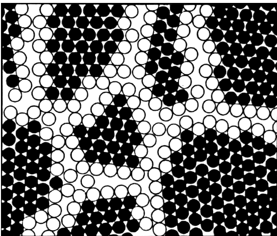
1. ábra • Nanokristályos anyag atomi szerkezete sematikus. Az üres körök a szemcsehatárokon lévő atomok.
