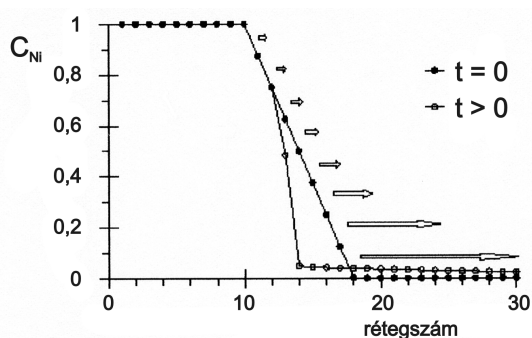
9. ábra • Eredetileg elmosódott határfelület kiélesedése (szimuláció Ni-Cu rendszerre).
